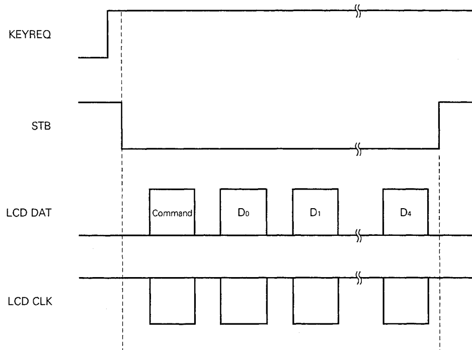
Fig. 4-4 Key Data Input/Output
