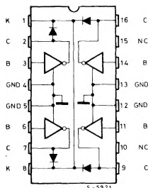
ULN2064B ULN2068B
