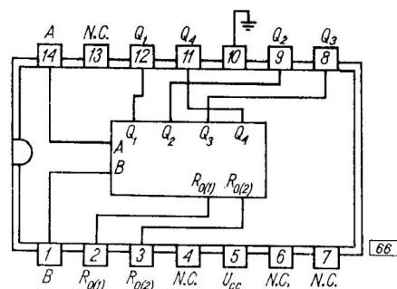
Rozkład wyprowadzeń (widok z góry) Czterobitowy licznik binarny
